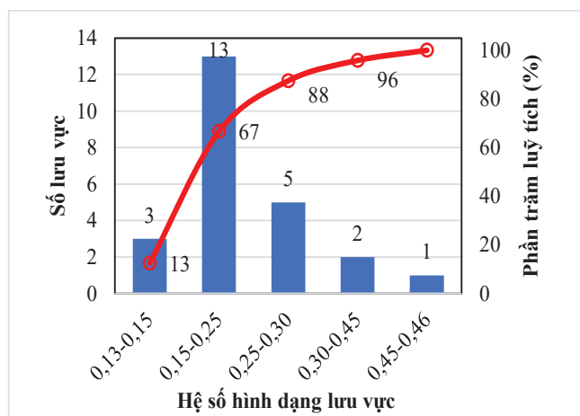
Hình 10. Biểu đồ quan hệ giữa số trận LBD và hệ số hình dạng lưu vực.
