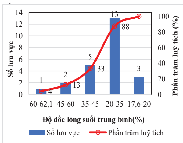
Hình 8. Biểu đồ quan hệ giữa số lưu vực LBD và độ dốc lòng suối trung bình.
