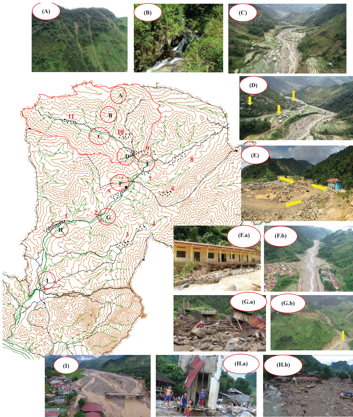
Hình 2. Một số hình ảnh điều tra thực địa về cơ chế tác động và thiệt hại do LBD năm 2017 và 2018. Các vị trí đánh số từ 1 đến 11 tương ứng với vị trí 11 bản bị thiệt hại của xã Nam Pao (1: Hua Nặm; 2: Huổi Liểng; 3: Nong Bâu; 4: Huổi Có; 5: Hốc; 6: Huổi Hốc; 7: Bâu; 8: Ít; 9: Piêng; 10: Huổi Sỏi; 11: Hua Piêng); (A) Xói lở bề mặt tạo rãnh xói ở khu phát sinh suối cấp 1 tại Nam Pao; (B) Khu vực dịch chuyển của LBD ở suối cấp 1 tại Huổi Lát và Nam Pao; (C) LBD mang theo nhiều đá vôi lấp toàn bộ ruộng và cuốn trôi nhà ven suối Piêng (chụp ảnh UAV tại vị trí Huổi Lát xã Nam Pao sau lũ 6 tháng); (D) Bản Piêng sau LBD (ảnh chụp sau lũ 6 tháng); (E) Trường Tiểu học Nam Pao nằm ở phía bờ cong lõm bị lũ phá hủy còn trơ lại 4 phòng học (ảnh chụp ngay sau lũ); (F.a) Trường học tại bản Hốc bị tàn phá trơ cả móng nhà (ảnh chụp ngay sau lũ); (F.b) Toàn cảnh từ vị trí UBND xã Nam Pao xuôi về hạ lưu sau lũ 6 tháng; (G.a) Nhà tại bản Huổi Liểng bị lũ phá hủy (ảnh chụp ngay sau lũ); (G.b) Nhà cửa của 16 hộ dân tại khu trũng tích bản Huổi Liểng bị cuốn trôi hoàn toàn; (H.a) Những người dân vô gia cư sau lũ (ảnh chụp ngay sau lũ); (H.b) Toàn cảnh bản Hua Nặm tan hoang sau lũ (ảnh chụp ngay sau lũ); (I) LBD xói lòng, bờ suối và cầu giao thông tại thị trấn Ít Ong (ảnh chụp ngay sau lũ).
